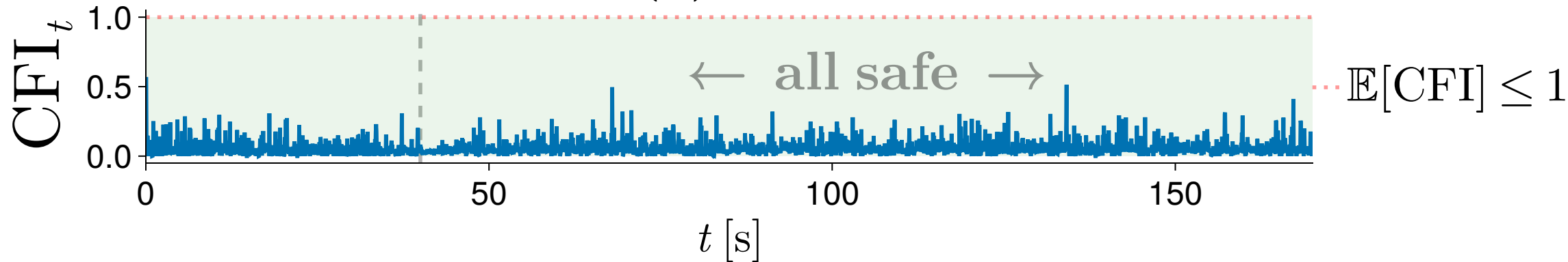
(d) \text{CFI}_t
